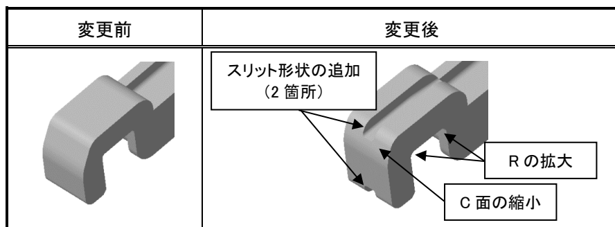
図 2. 可接キャリア形状の変更について
